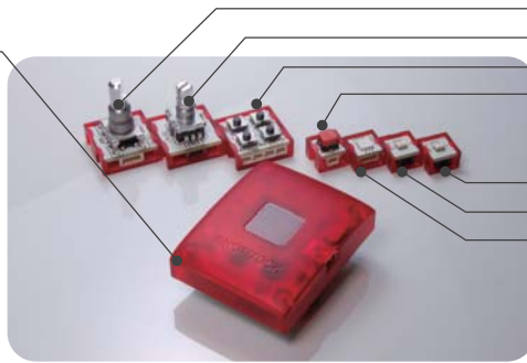
コアユニット 43x53x12.7mm デバイス大 22x22x7.9mm デバイス小 12x12x7.9mm
